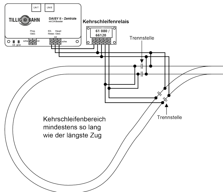
Anschlusskizze eines Kehrschleifenrelais
