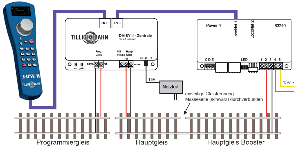
Anschlusskizze eines Boosters
