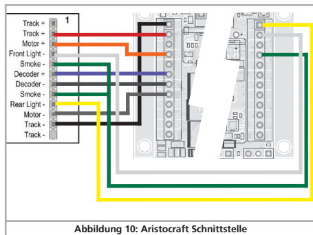
Abbildung 10: Aristocraft Schnittstelle
