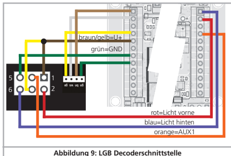
Abbildung 9: LGB Decoderschnittstelle
