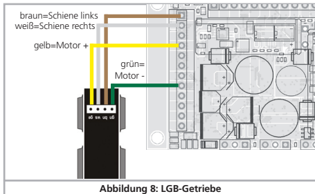
Abbildung 8: LGB-Getriebe
