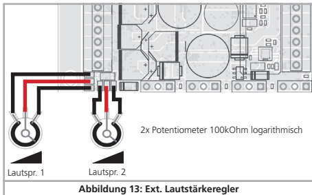
Abbildung 13: Ext. Lautstärkereglер
