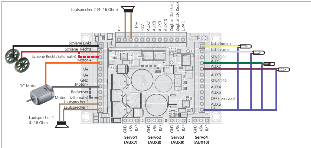
Abbildung 7: Allgemeines Anschlussschema LokSound XL V4.0 (Beispielverdrahtung)
